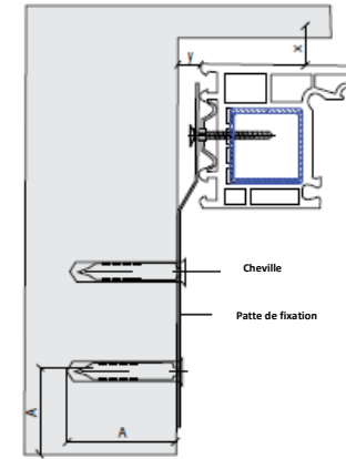
Fig.2 Installation du cadre de la fenêtre sur la cheville.
